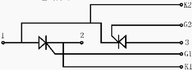
电路图
